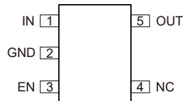
SOT23-5 SC70-5
