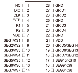
SOP28
